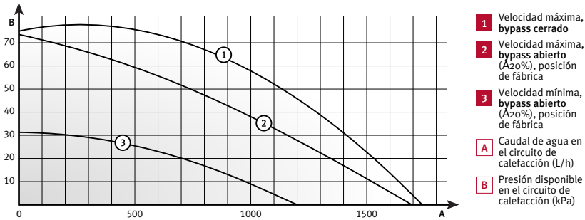
Curva de presión disponible de la bomba del circuito de calefacción Isofast Condens de 35 kW
